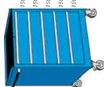
● h. 980 mm • 5 cassetti MR85 04 estrazione parziale MR85 04T estrazione totale 200 kg MR85 04V estrazione totale 75 kg
