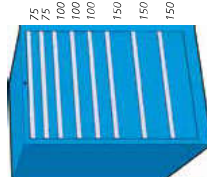
● h. 1000 mm • 8 cassetti M100 05 estrazione parziale M100 05T estrazione totale 200 kg M100 05V estrazione totale 75 kg
