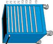
● h. 980 mm • 8 cassetti MR85 03 estrazione parziale MR85 03T estrazione totale 200 kg MR85 03V estrazione totale 75 kg
