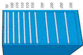
● h. 1450 mm • 10 cassetti M145 101 estrazione parziale M145 101T estrazione totale 200 kg M145 101V estrazione totale 75 kg
