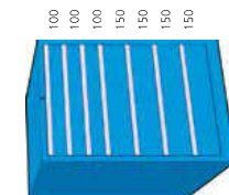
● h. 1000 mm • 7 cassetti M100 73 estrazione parziale M100 73T estrazione totale 200 kg M100 73V estrazione totale 75 kg
