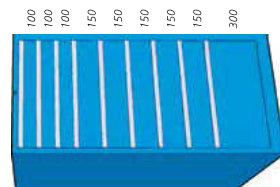
● h. 1450 mm • 9 cassetti M145 92 estrazione parziale M145 92T estrazione totale 200 kg M145 92V estrazione totale 75 kg
