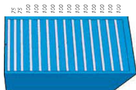
● h. 1450 mm • 14 cassetti M145 114 estrazione parziale M145 114T estrazione totale 200 kg M145 114V estrazione totale 75 kg
